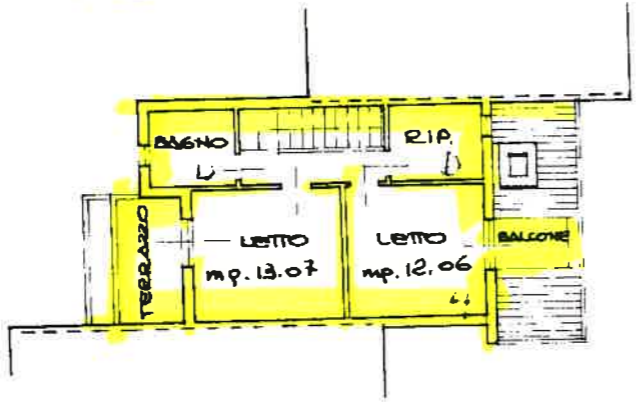
PIANO SECONDO h=2,80
